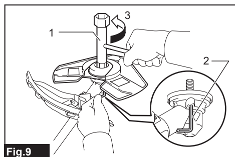
Fig.9 ► 1. Clé à douille 2. Clé hexagonale 3. Serrer
