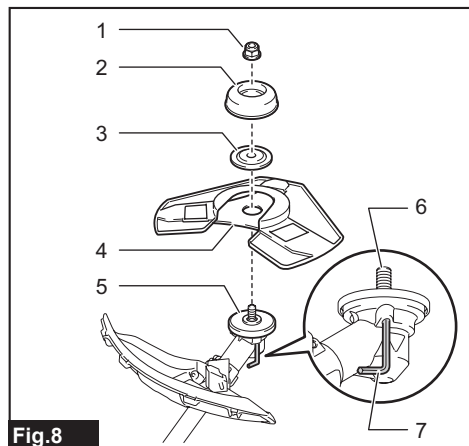
Fig.8 ► 1. Écrou 2. Coupelle 3. Rondelle de serrage 4. Lame de métal 5. Rondelle d'appui 6. Arbre 7. Clé hexagonale
